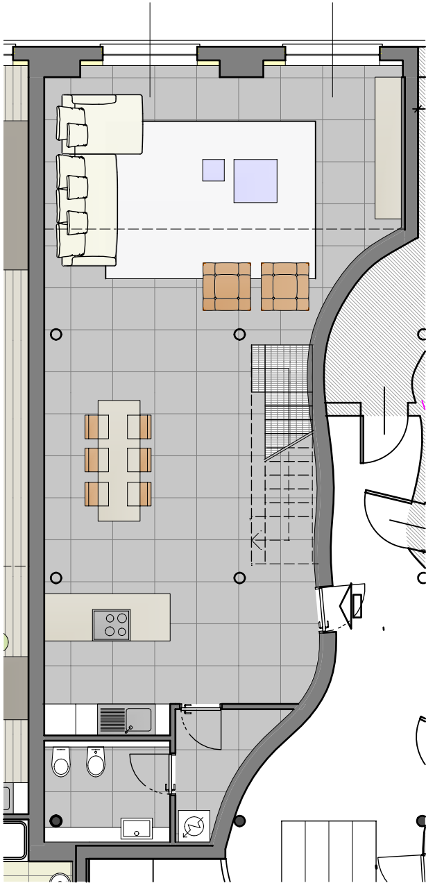
PIANO SECONDO
